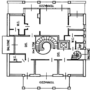
PIANTA PIANO PRIMO 1\200
