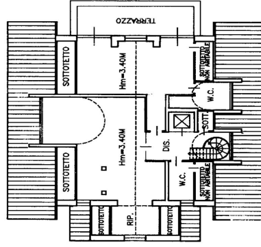
PIANTA PIANO SOTTOTETTO 1\200
